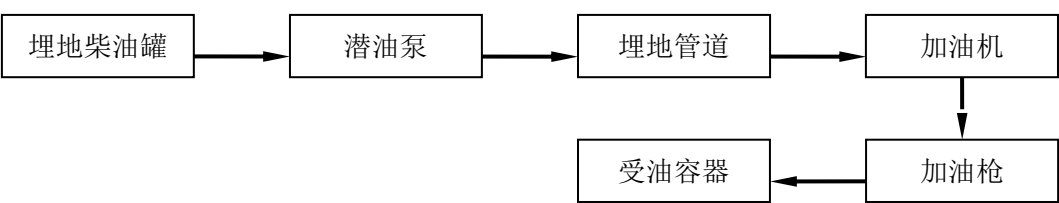
图 2.4-4 柴油加油工艺流程图示意简图
