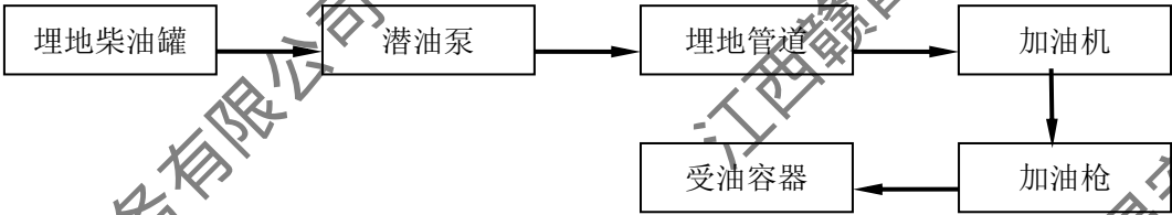
图 2.5-4 柴油加油工艺流程图示意简图 7
